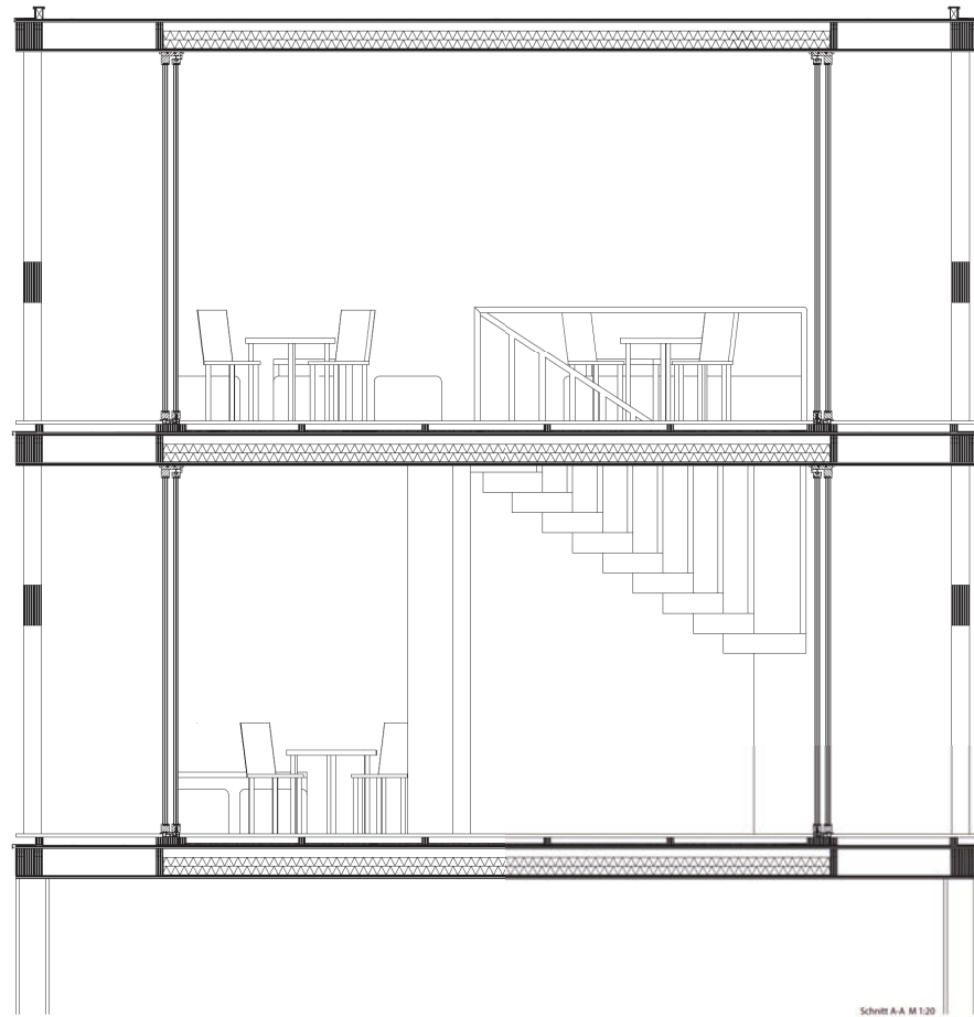
Schnitt AA M 1:20
