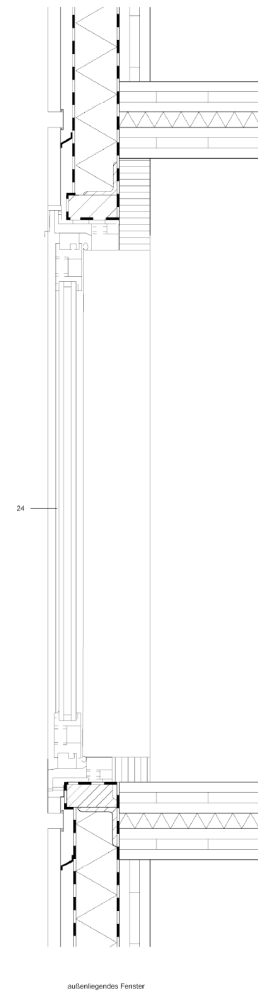
außenliegendes Fenster
